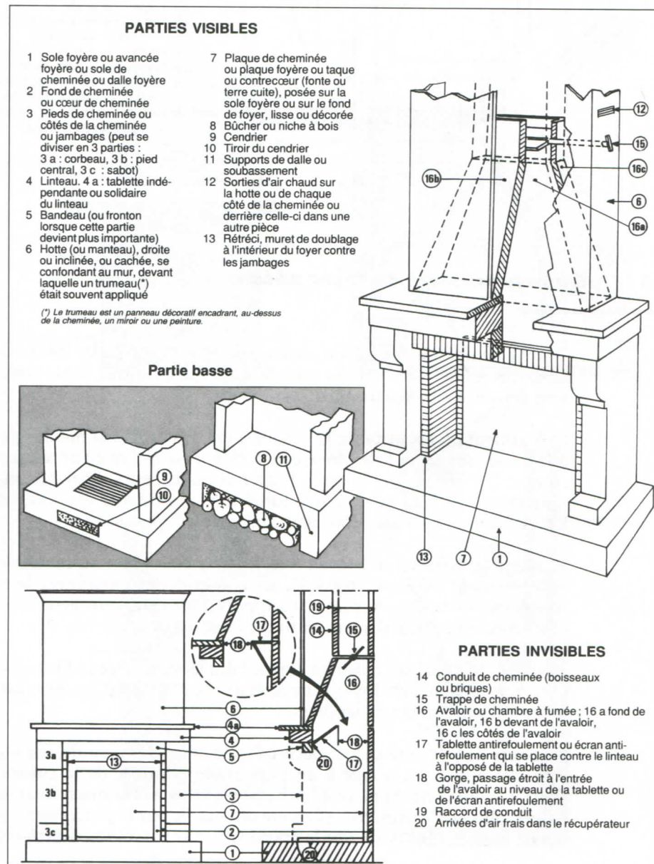
Figure 4.1 – Anatomie d'une cheminée.
