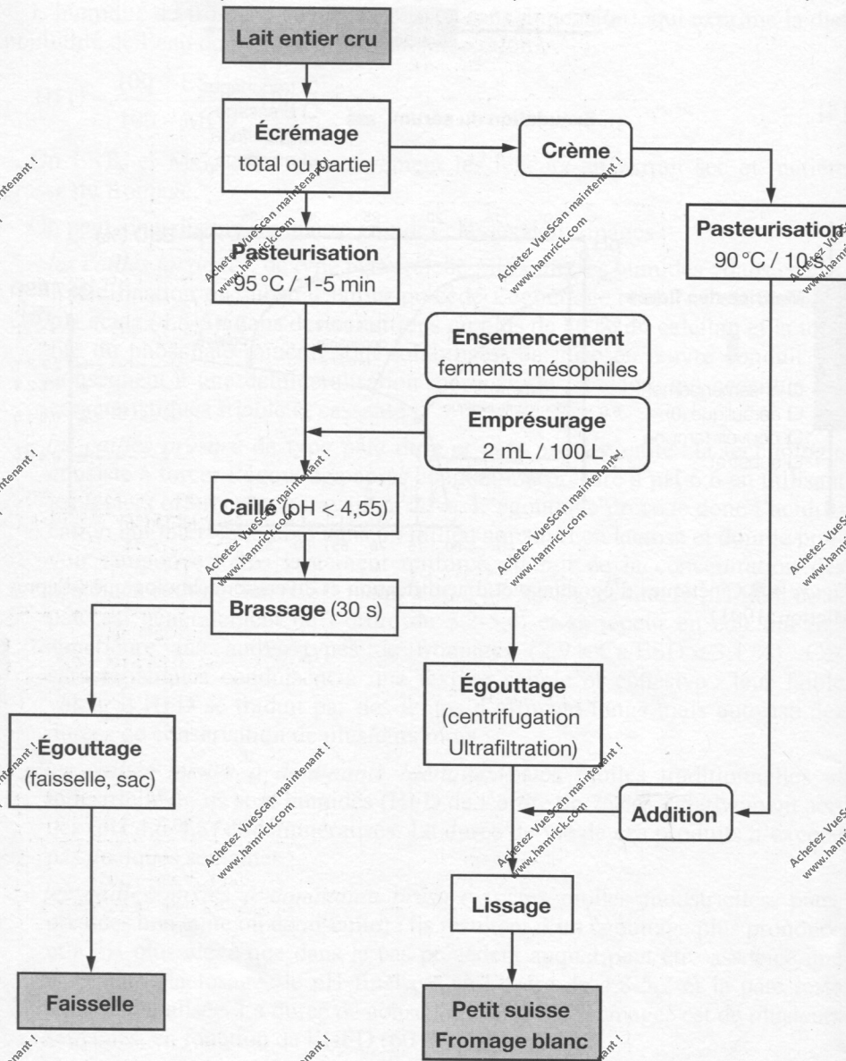
Figure 5 ■ Schéma général de la technologie de fabrication des fromages frais.
